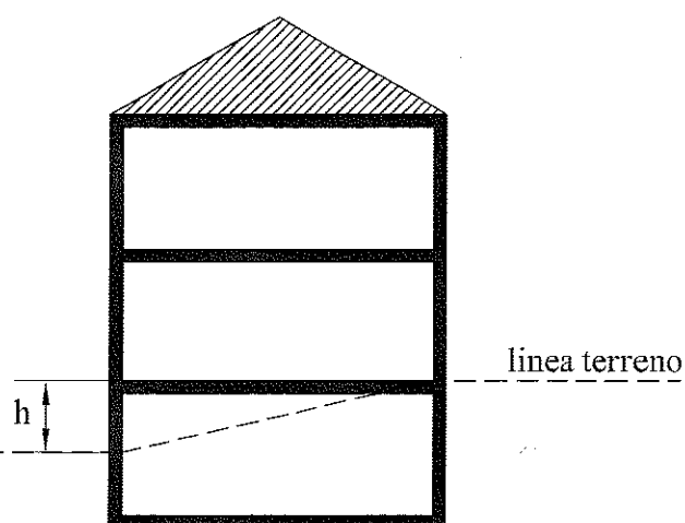
d) n° 2 piani di costruzione se h \leq 1.20 m n° 3 piani di costruzione se h > 1.20 m
